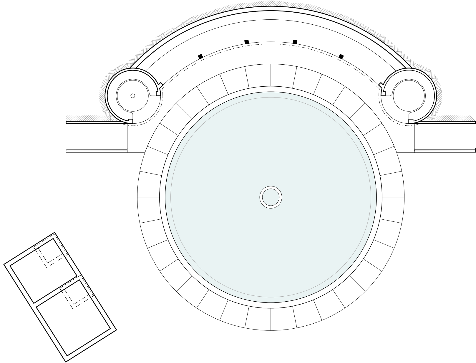
Grundriss
