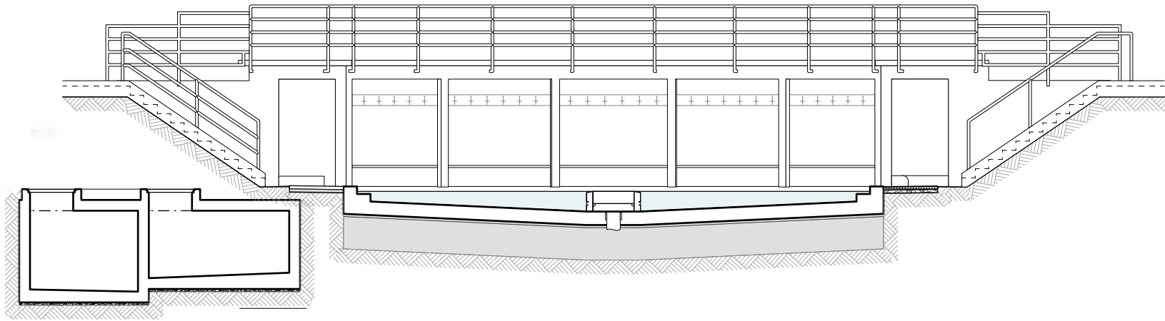
Querschnitt
