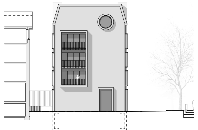
Stirnfassade zum Park
