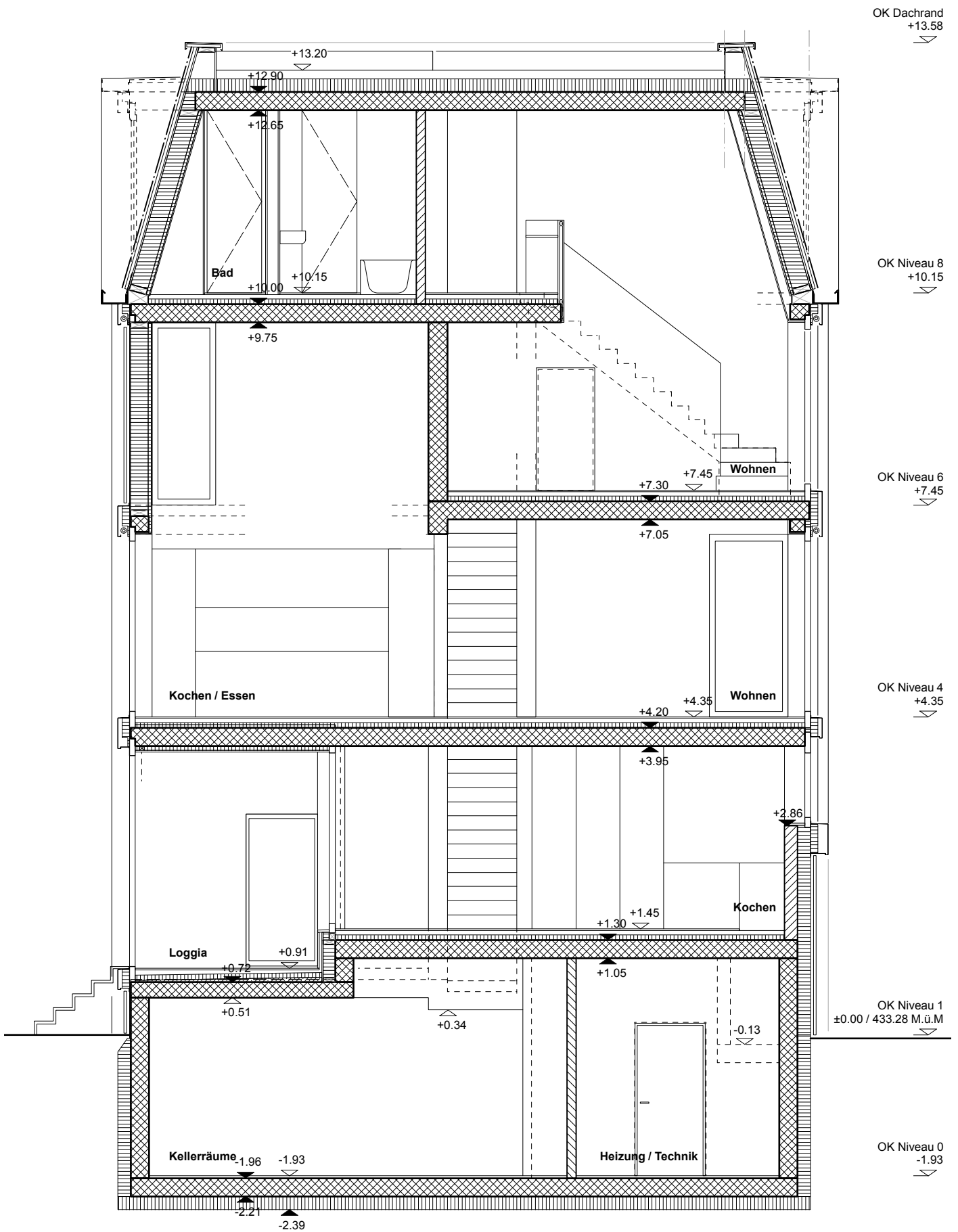
Konstruktionsschnitt
