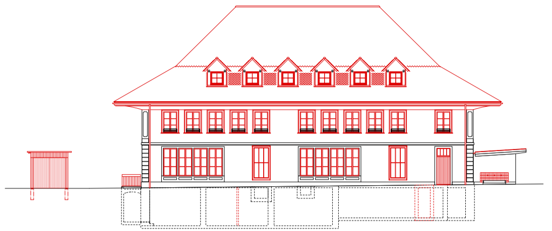
Südfassade
