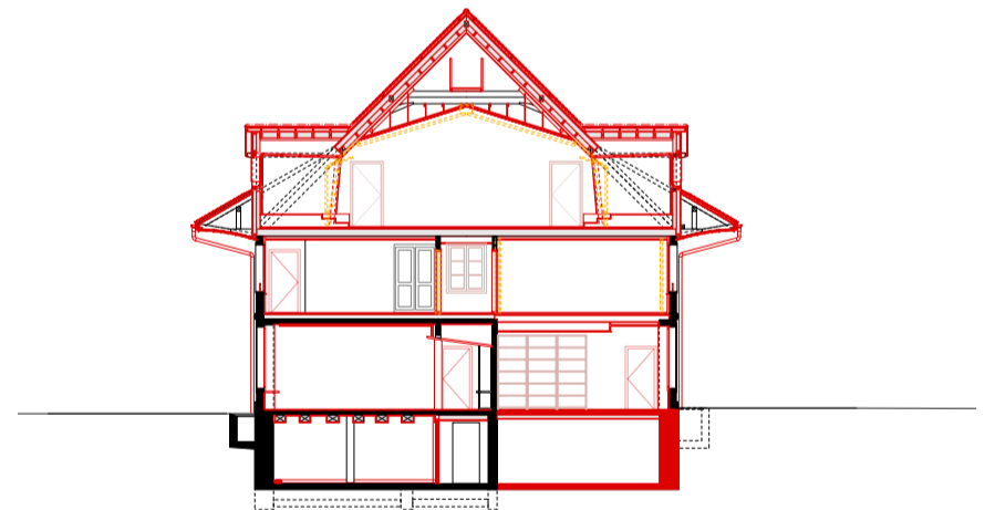
Querschnitt durch Lukarne
