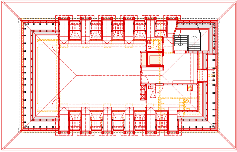
Grundriss Dachgeschoss
