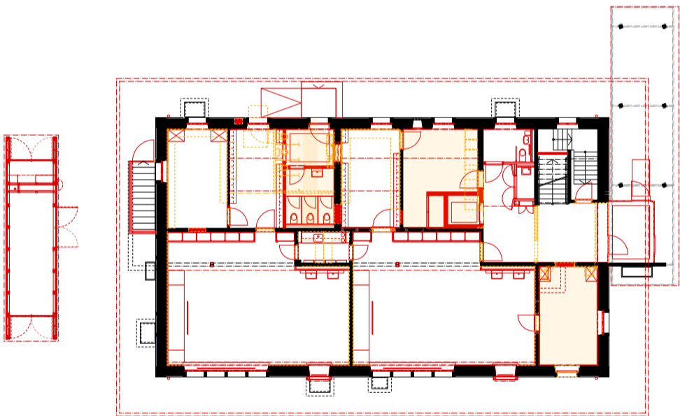
Grundriss Eingangsgeschoss
